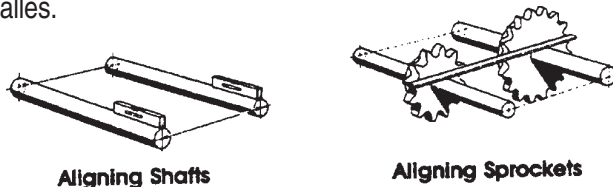
Figura 27. Eje y alineamiento de la catarina de impulso
