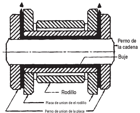
Figura 29. Sección cruzada de los eslabones de la cadena
