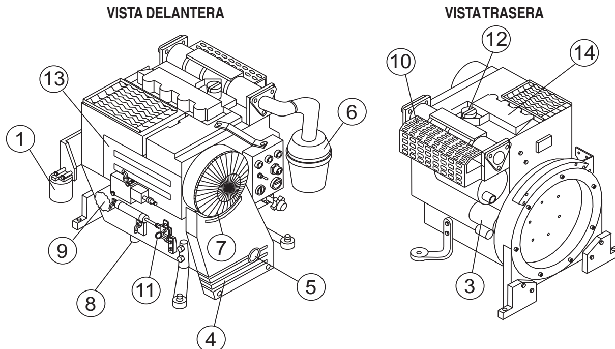
Figura 8. Componentes principales del motor modelo Deutz F2L01011F
