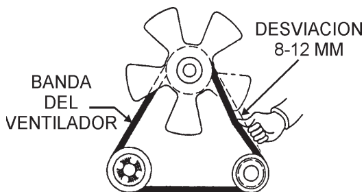
Figura 15. Desviación de la banda-V
