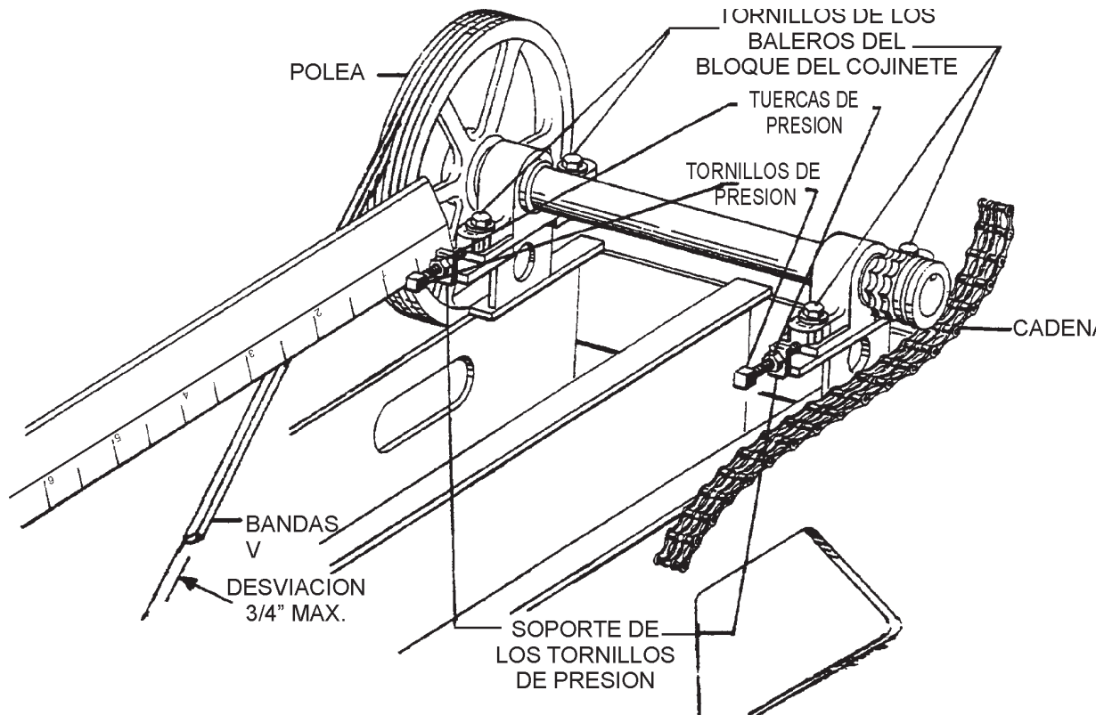
Figura 25. Banda-V y el ajuste de la cadena de impulso
