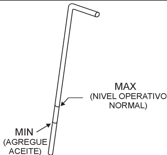
Figura 16. Varilla medidora de la caja de lubricación
