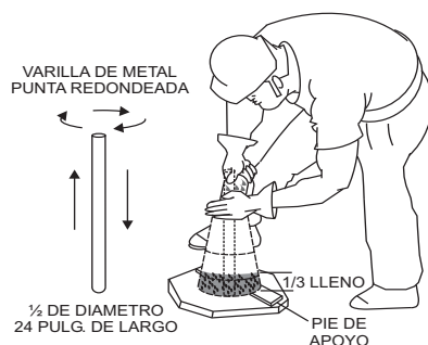
Figura 32-A. Prueba de asentamiento (1/3 de lleno)
