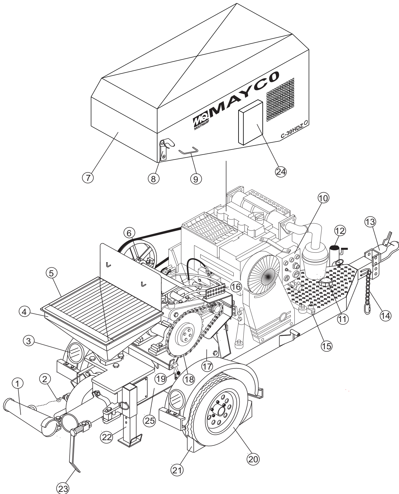
Figura 6. Componentes principales de la bomba
