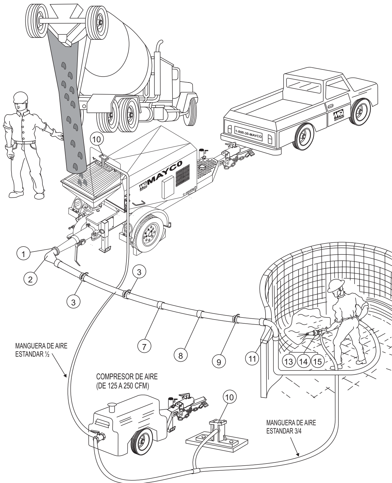
Figura 33. Sistema de tira concreto
