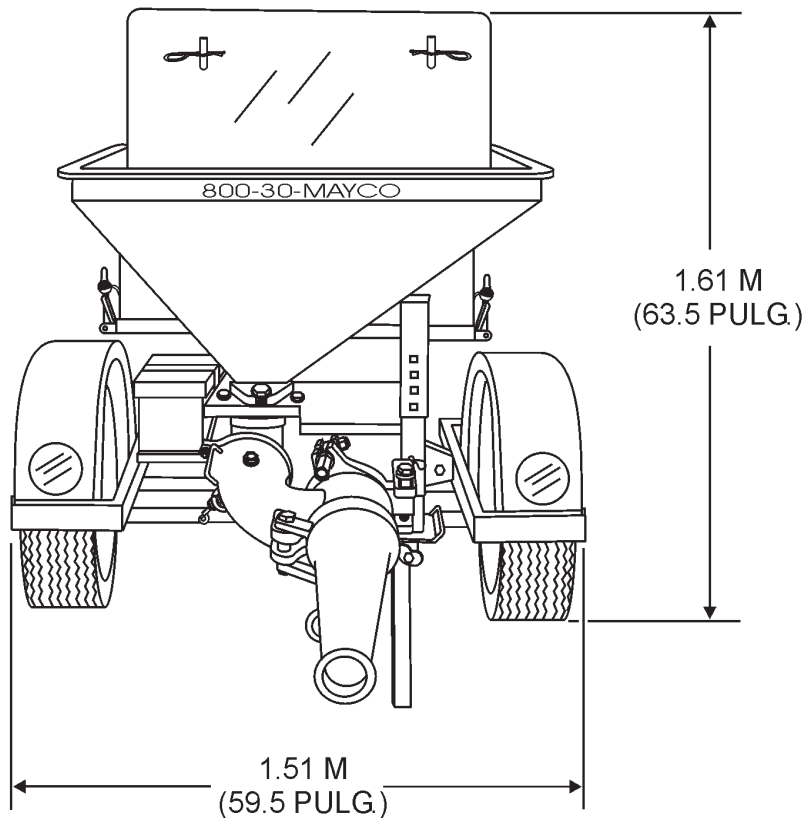
Figura 1. Dimensiones de la bomba de concreto C-30HDZ
