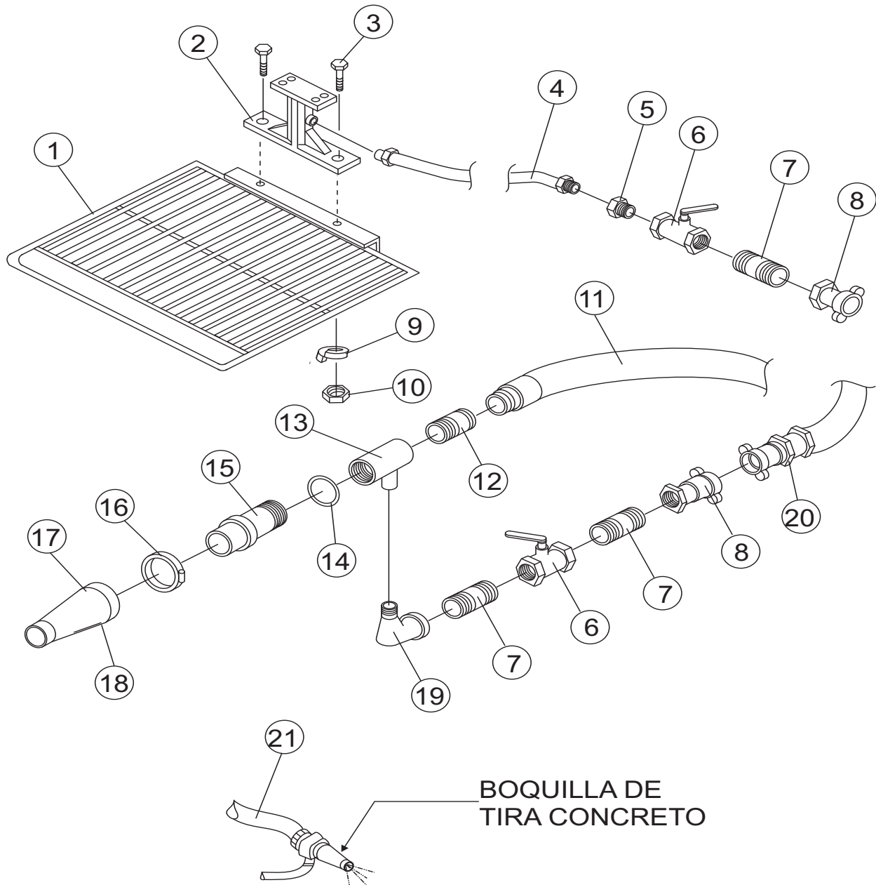
Figura 34. Accesorios del sistema de tira concreto
