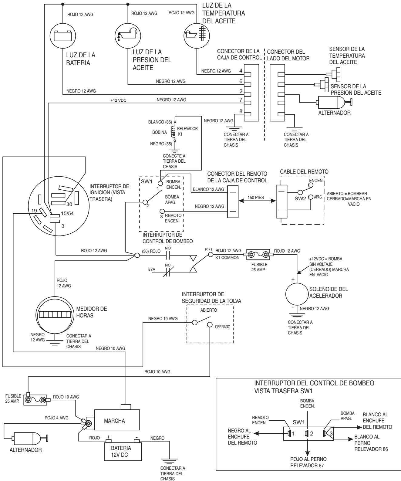
Figure 30. Diagrama del cableado
