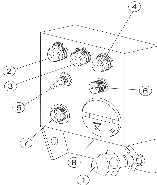
Figura 7. Componentes de la caja de control
