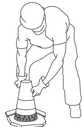
Figura 32-E. Prueba de asentamiento (Cono invertido)
