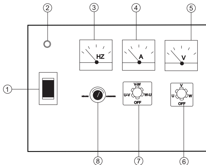
Figure 4. Panneau de Commande du Générateur
