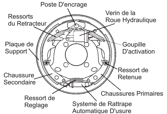
Figure 55. Composants du Frein Hydraulique
