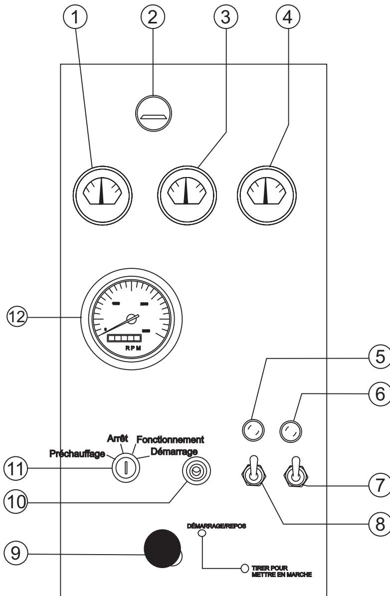
Figure 5. Panneau de Fonctionnement du Moteur
