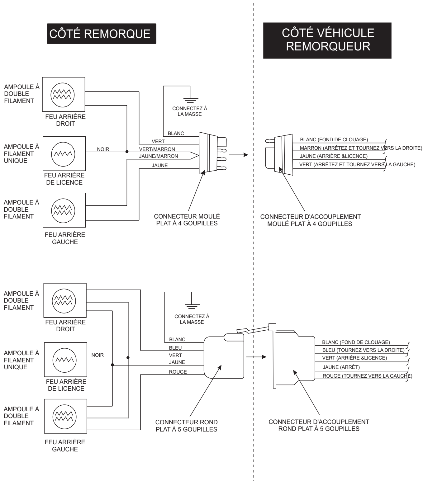
Figure 58. Schéma de Câblage du Véhicule de Remorquage/de la Remorque
