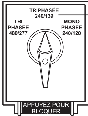
Figure 22. Commutateur de Sélection de la Tension 240/139 V Position Triphasée
