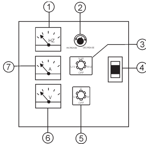
Figure 4. Panneau de Commande du Générateur
