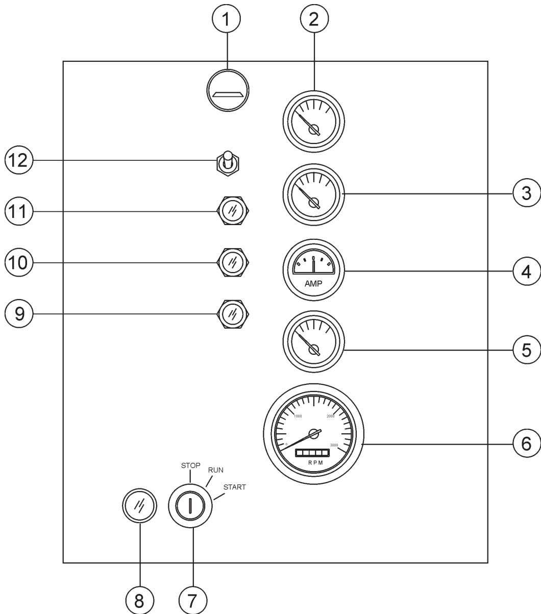
Figure 5. Panneau de Fonctionnement du Moteur
