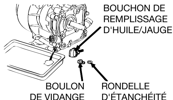
Schéma 27. Vidange d'huile moteur
