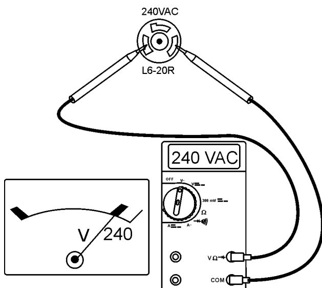
Schéma 20. Prise 240V
