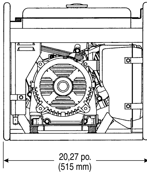
Schéma 1. Dimensions
