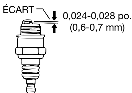
Schéma 26. Écartement des bougies d'allumage
