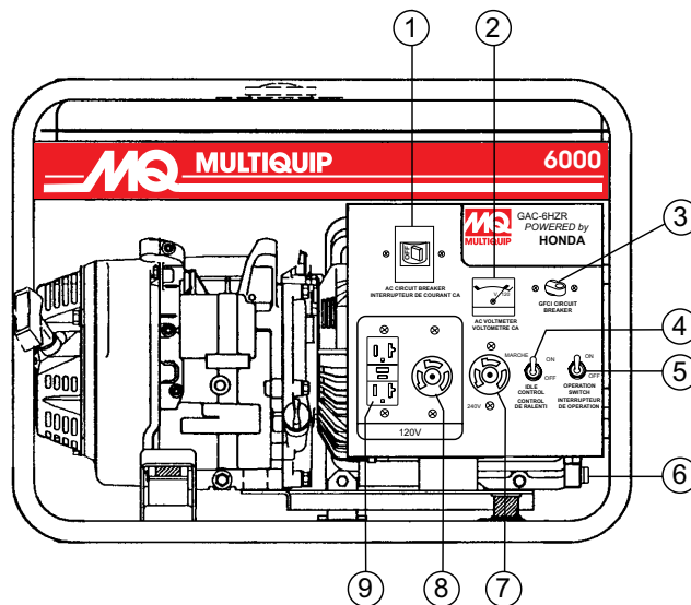
Schéma 3. Composants de générateur
