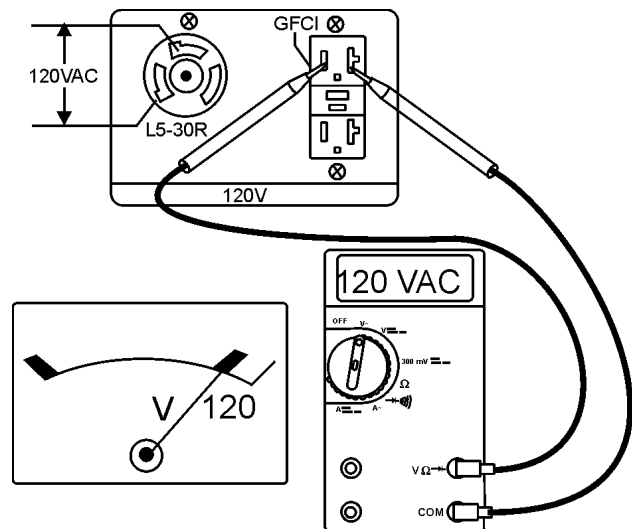
Schéma 19. Prises 120V/disjoncteur différentiel
