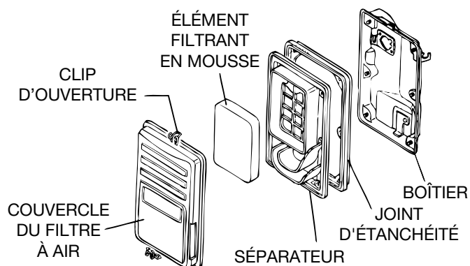
Schéma 28. Filtre à air du moteur
