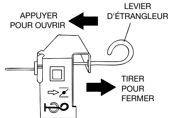
Schéma 12. Levier d'étrangleur
