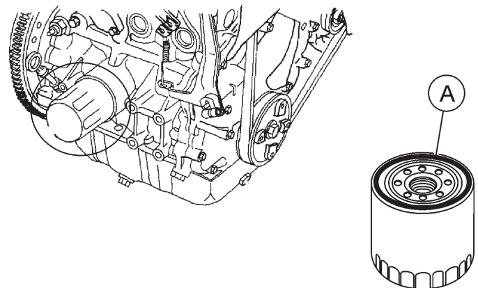
Rys. 15 Filtr olejowy
