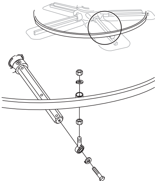
Figure 34. Pierścień stabilizujący
