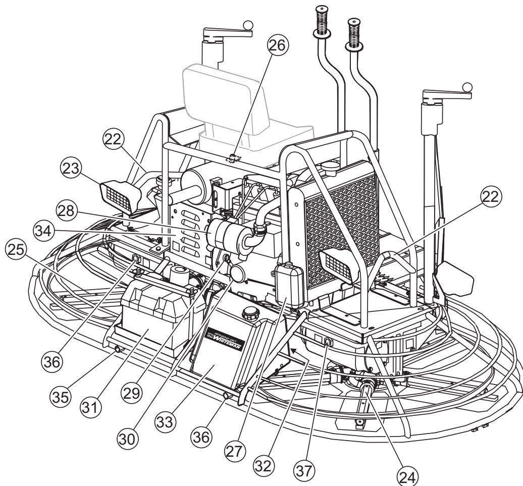
Figura 4. HHN-31V Controles e indicadores (Vista trasera)
