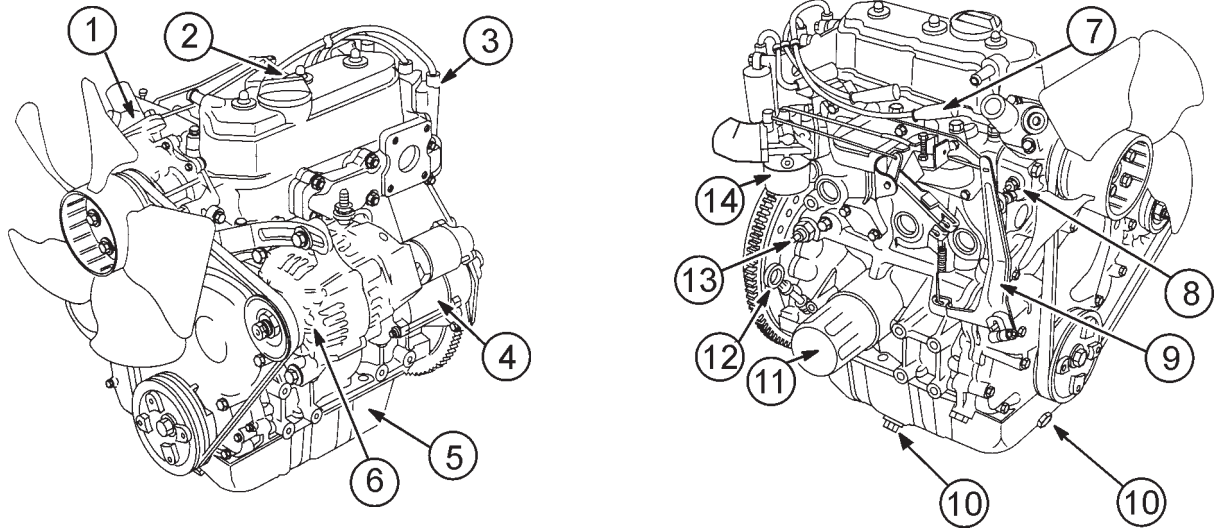
Figura 5. Controles y componentes del motor a gasolina
