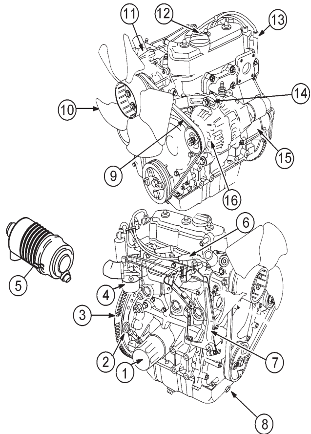
Figura 13. Areas de servicio del motor
