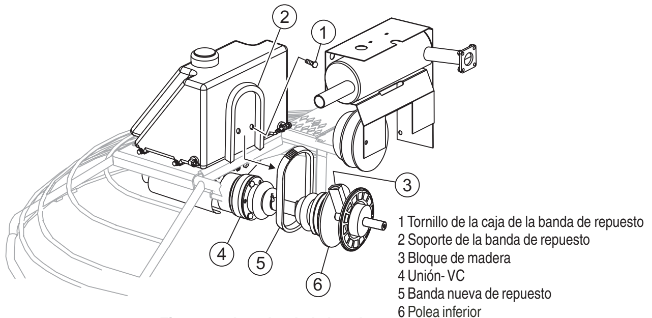
Figura 20. Instalando la banda
