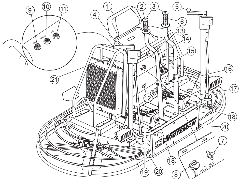
Figura 3. Controles e indicadores HHN-31V (Vista delantera)
