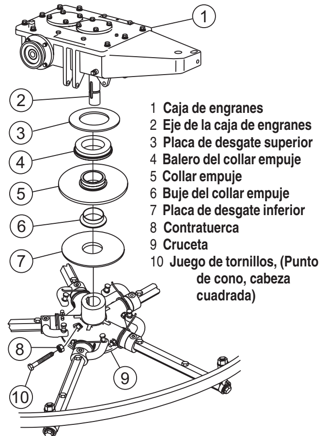
Figura 32. Retiro de la cruceta/caja de engranes
