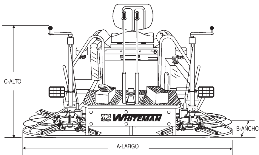
Figura 2. Especificaciones de las dimensiones de la HHN-31V
