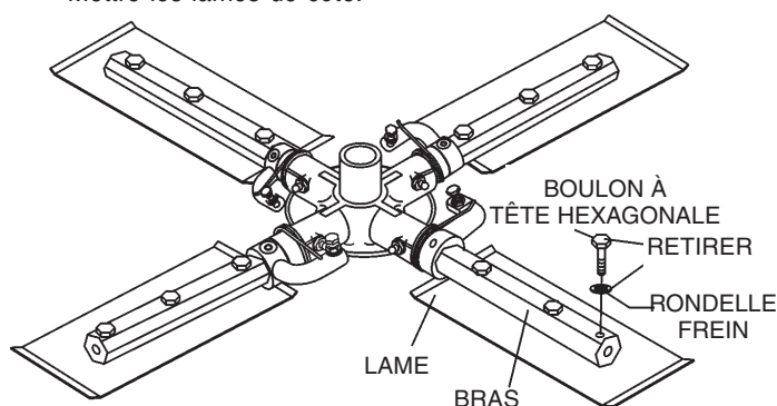
Figure 24. Lames de truelle
