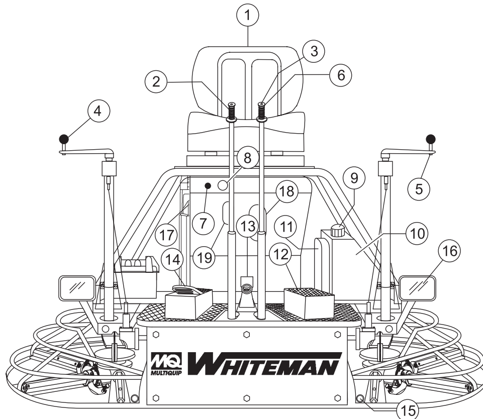
Figure 5. Commandes et indicateurs JTO (avant)
