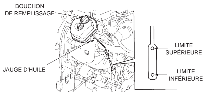
Figure 7. Jauge d'huile de moteur
