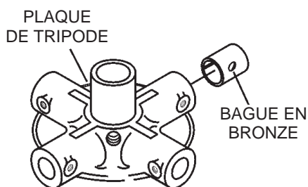
Figure 23. Bagues en bronze
