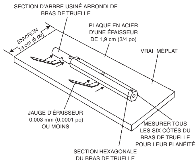
Figure 25. Test de planéité de bras de truelle
