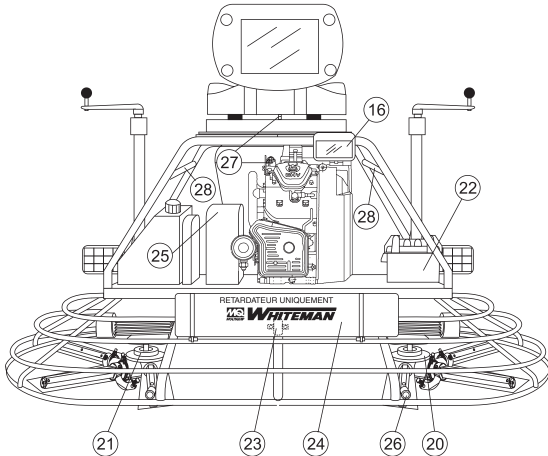
Figure 6. Commandes et indicateurs JTO (arrière)
