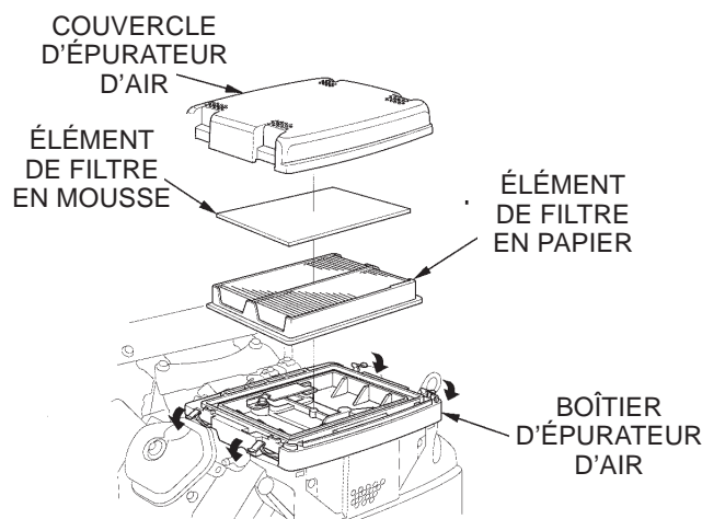
Figure 14. Épurateur d'air
