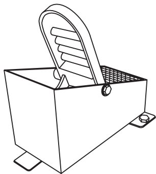
Figure 9. Pédale de commande de vitesse des lames
