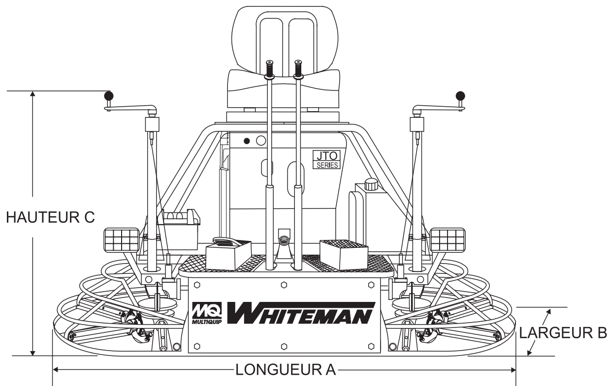
Figure 2. Dimensions de la truelle
