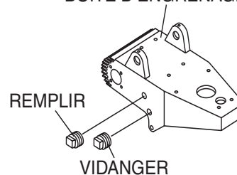
Figure 8. Bouchons d'huile de boîte d'engrenage
