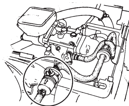
Figure 16. Filtre à carburant
