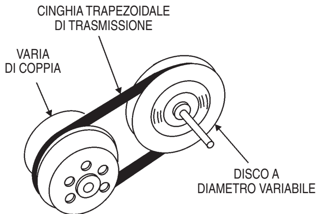
Figura 21. Variatore di coppia/Puleggia a diametro variabile
