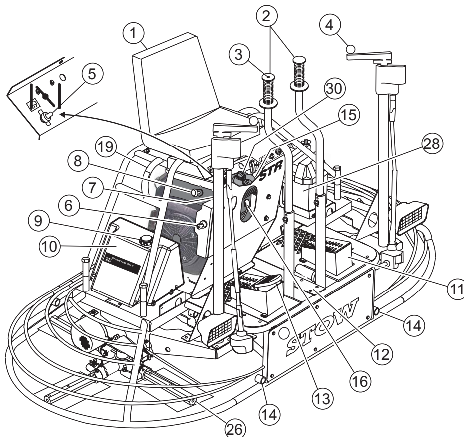
Figura 2. Comandi e indicatori della serie STR36 (vista frontale)
