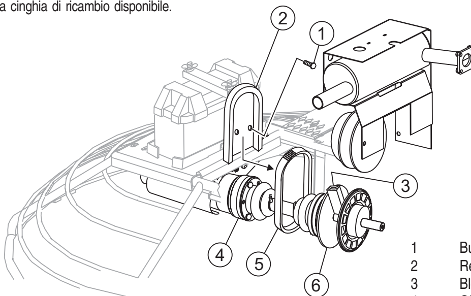
Figura 19. Installazione della cinghia di trasmissione
