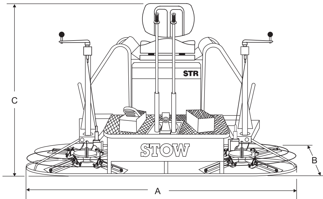
Figura 1. Dimensioni della frattazzatrice meccanica SERIE STR36
