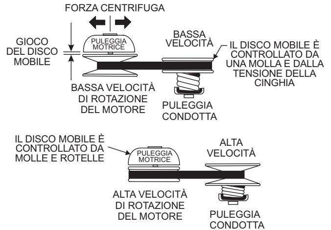
Figura 23. Interazione delle pulegge
