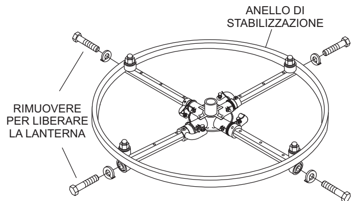
Figura 30. Anello di stabilizzazione
