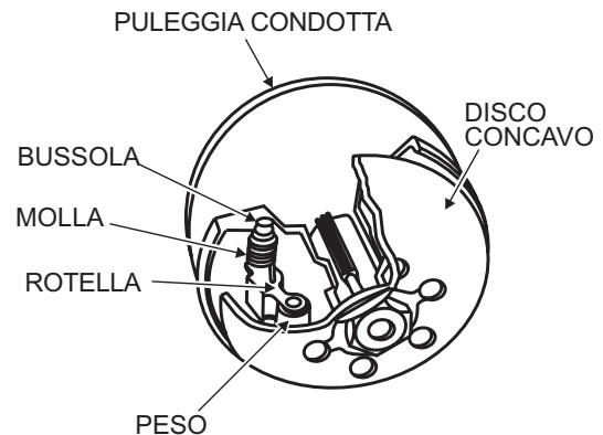
Figura 24. Puleggia a diametro variabile
