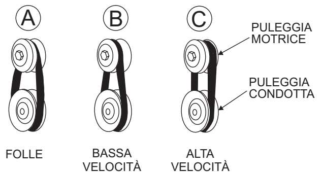
Figura 25. Condizioni delle pulegge
