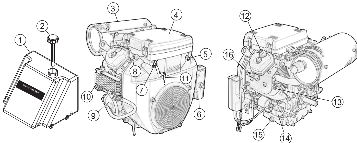
Figura 4. Comandi e componenti del motore
