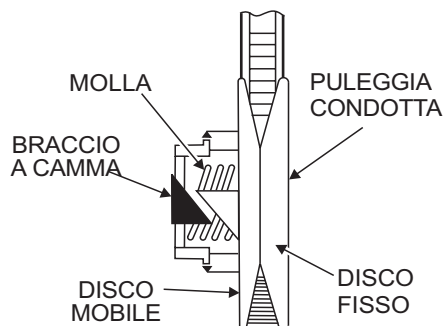
Figura 26. Molla e braccio a camma della puleggia
