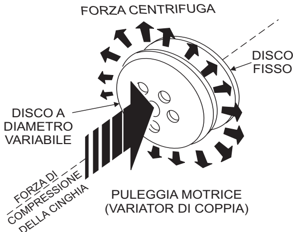
Figura 22. Variatore di coppia (forza centrifuga)
