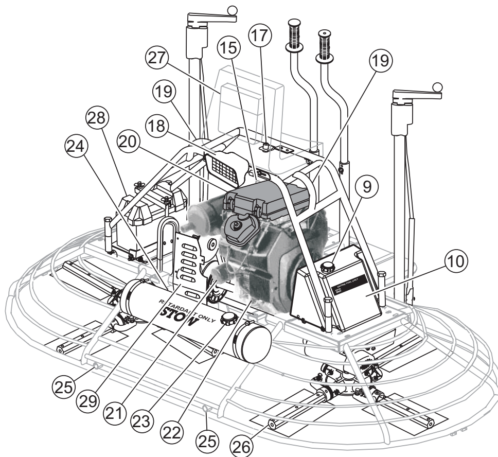
Figura 3. Comandi e indicatori della SERIE STR36 (vista posteriore)
