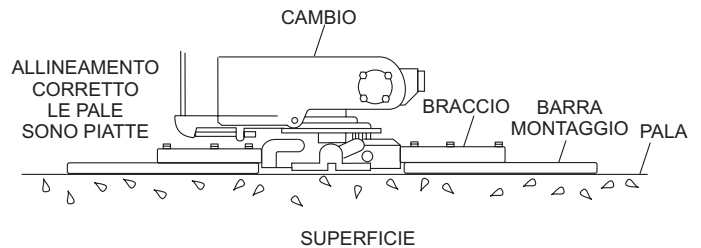
Figura 29. Allineamento corretto della flangia della lanterna
